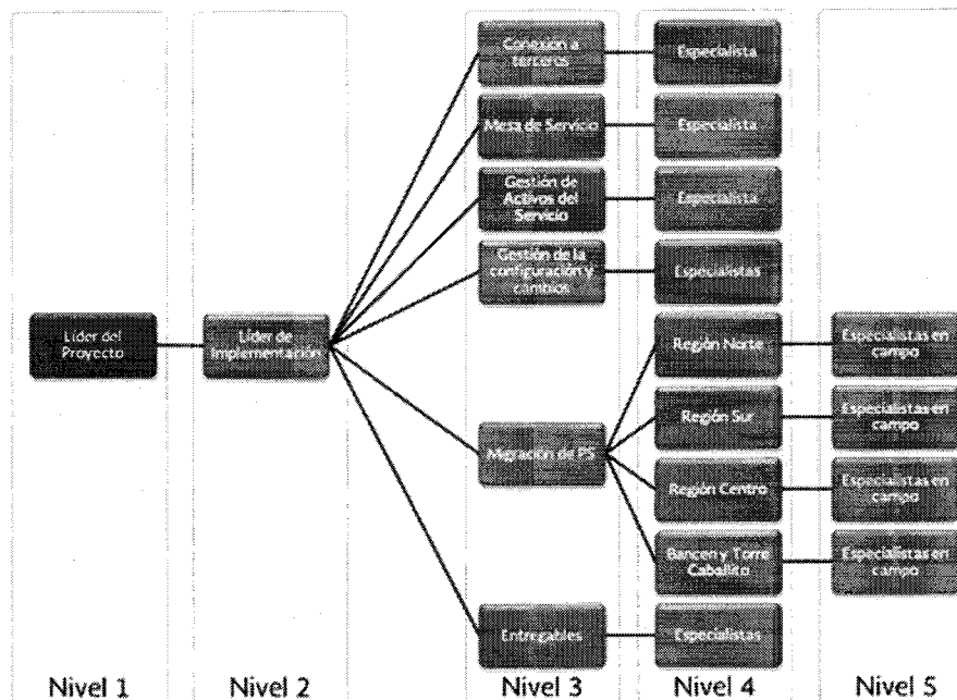
Diagrama 22: Implementación
