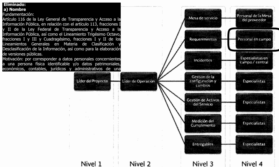
Diagrama 23: Operación
