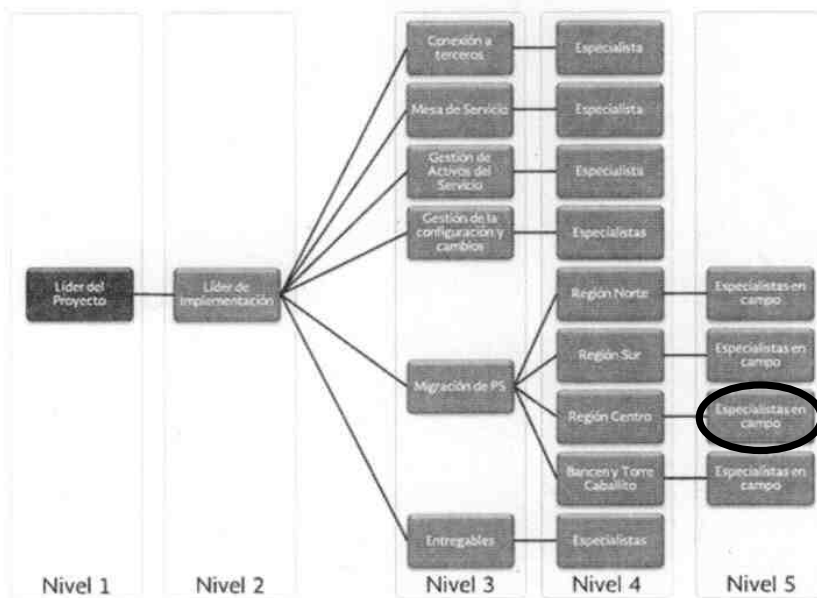
Diagrama 22: Implementación
