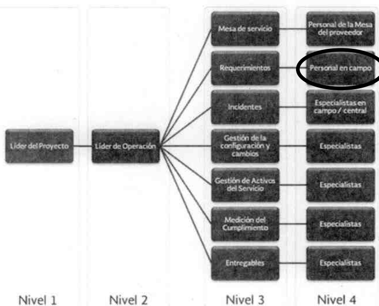
Diagrama 23: Operación
