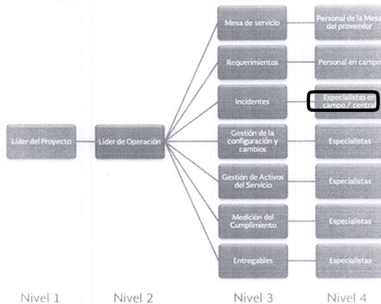
Diagrama 23: Operación
