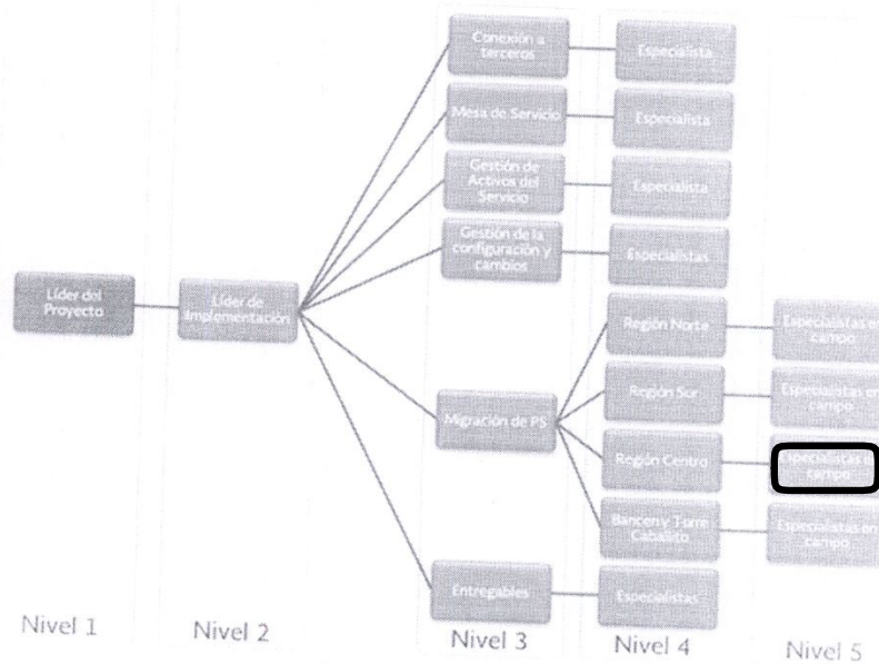
Diagrama 22: Implementación
